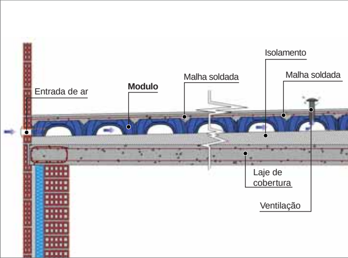
Exemplo de telhado ventilado
